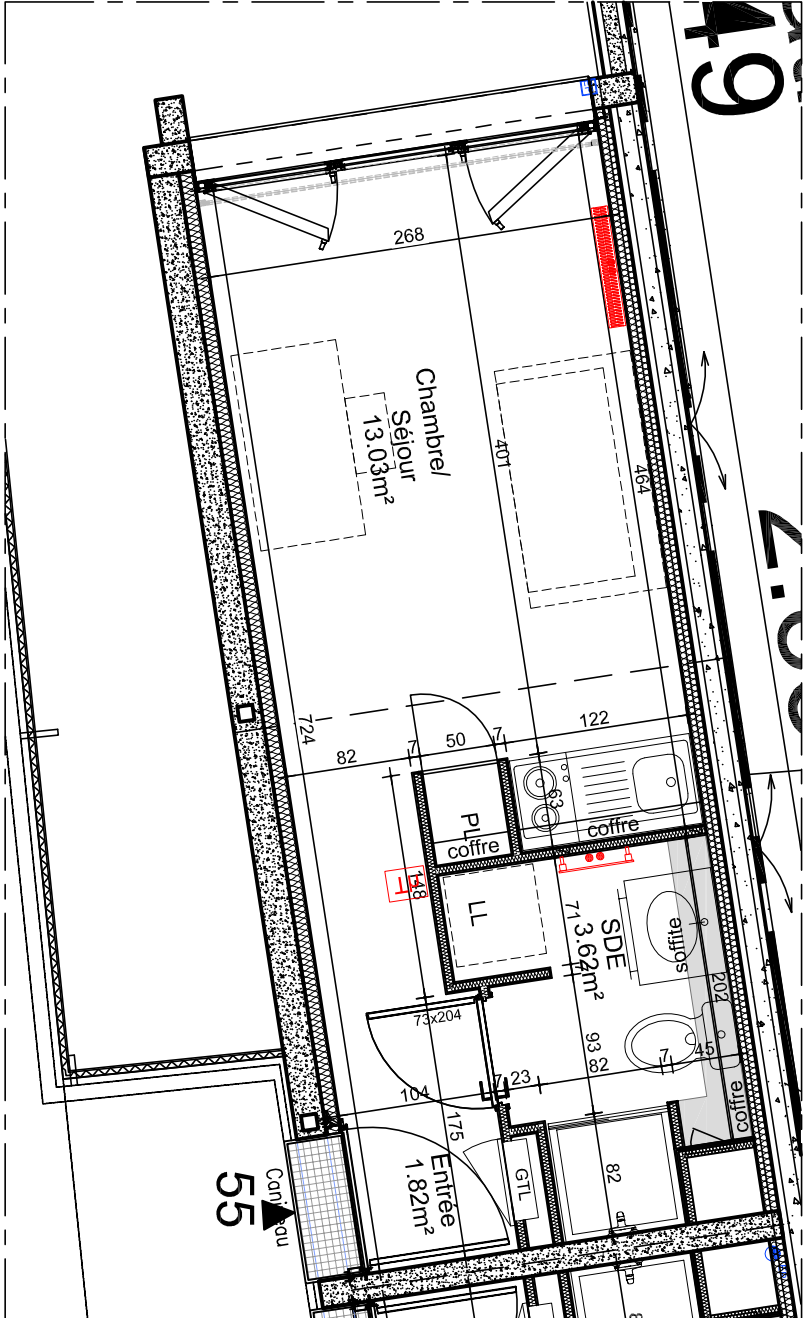
PLAN R+2
